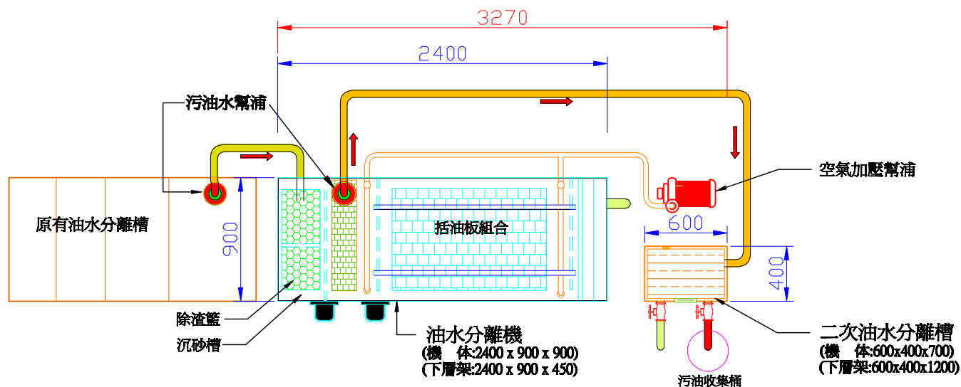
俯視圖
